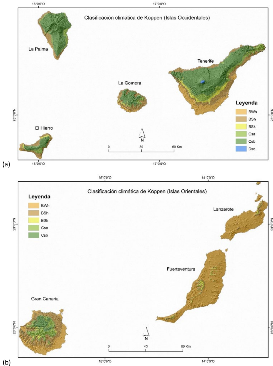
Figura 5.1 Mapas de clasificación climática de Köppen (a) Islas occidentales, (b) Islas Orientales
