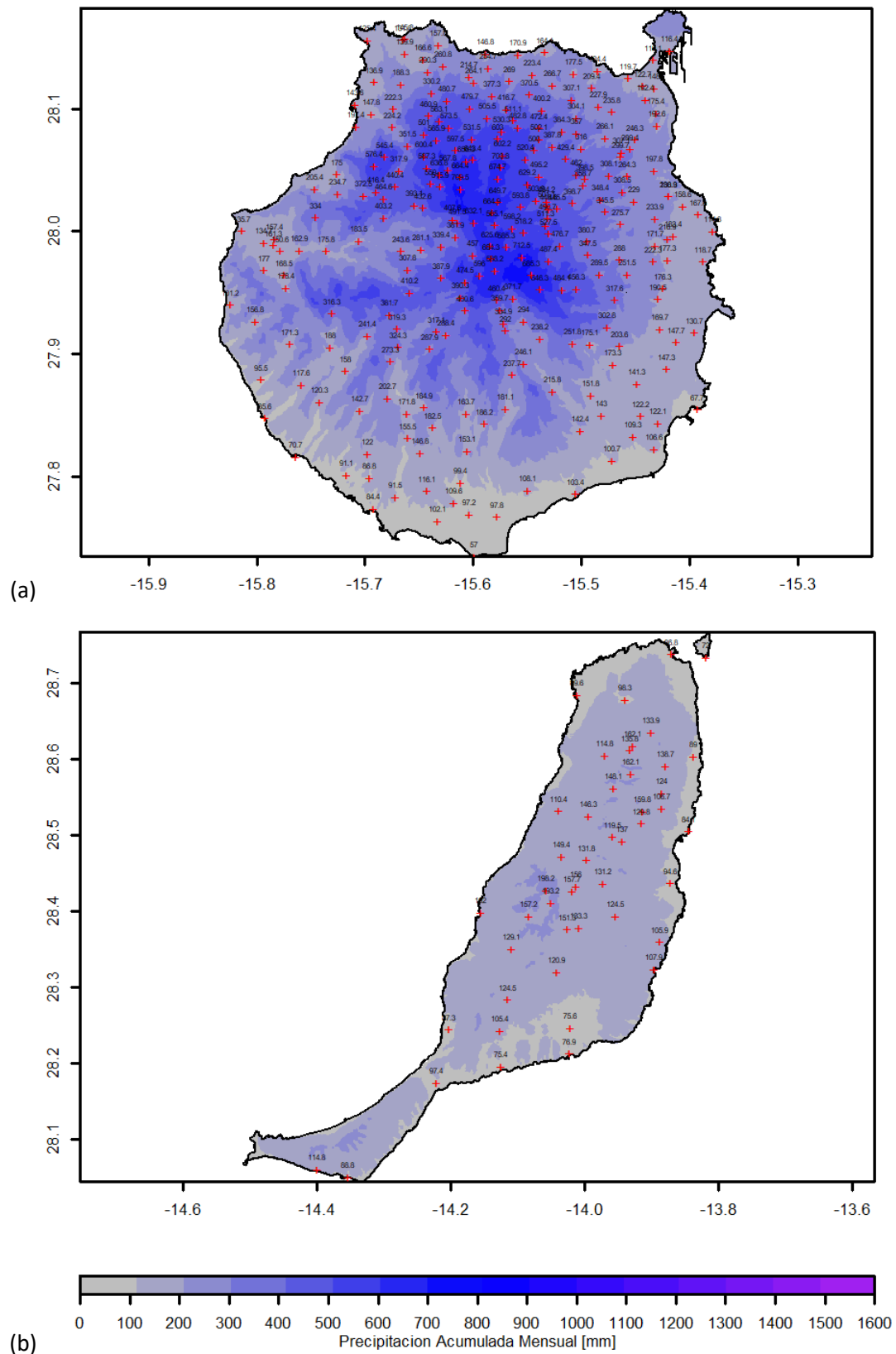
Figura 4.2.2. Precipitación acumulada anual en mm a 100 m de resolución espacial promediados para el periodo 1970-2020. (a) Isla de Gran Canaria, (b) Isla de Fuerteventura. Las cruces indican las posiciones de las estaciones meteorológicas utilizadas y los valores numéricos son las acumulaciones promediadas de cada estación.
