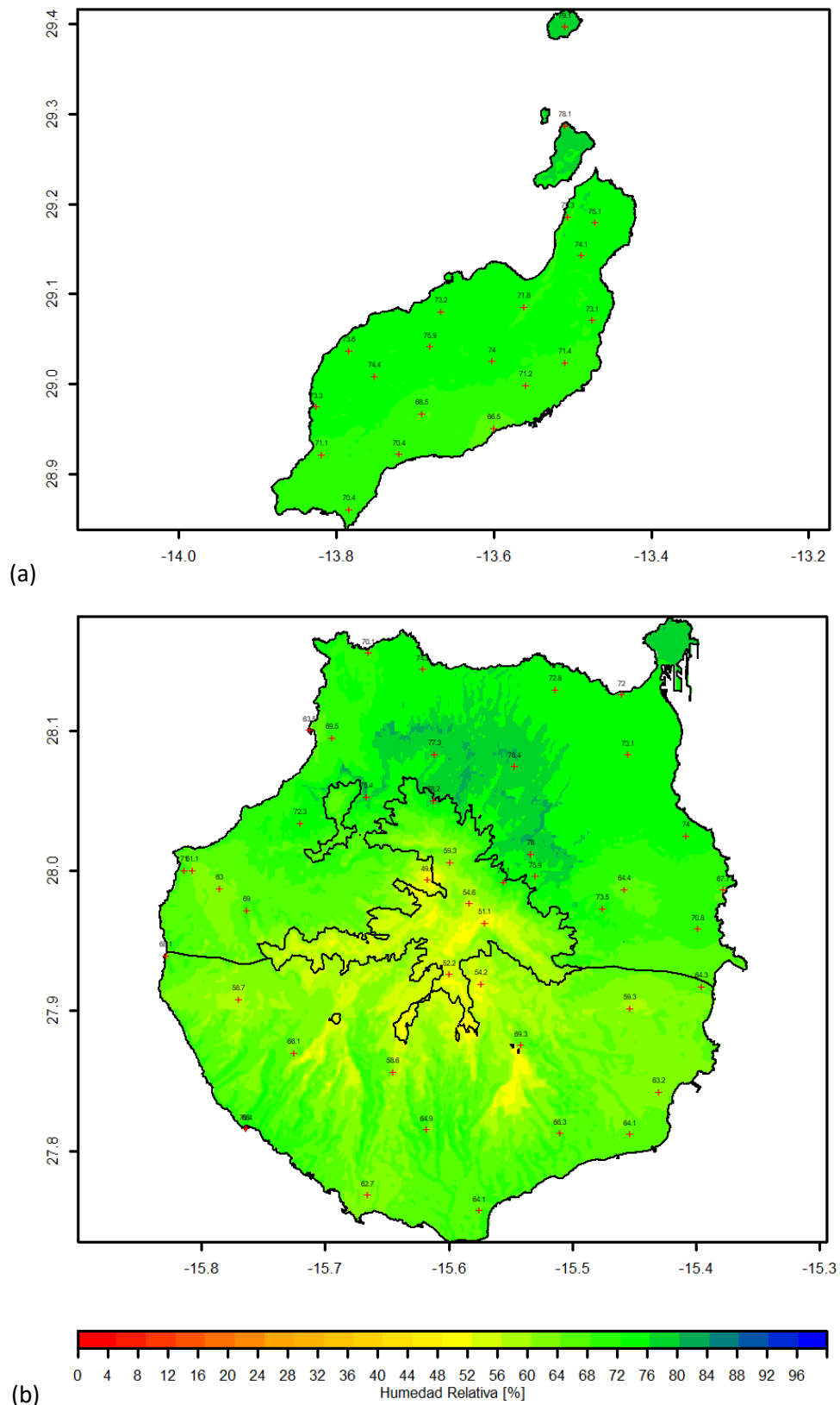
Figura 4.3.3. Humedad relativa a 100 m de resolución espacial promediados para el periodo 1991-2018 para la isla de Lanzarote (a) y entre 1991-2020 para la Isla de Gran Canaria (b). Las cruces indican las posiciones de las estaciones meteorológicas utilizadas y los valores numéricos son los valores promediados de las humedades de cada estación.
