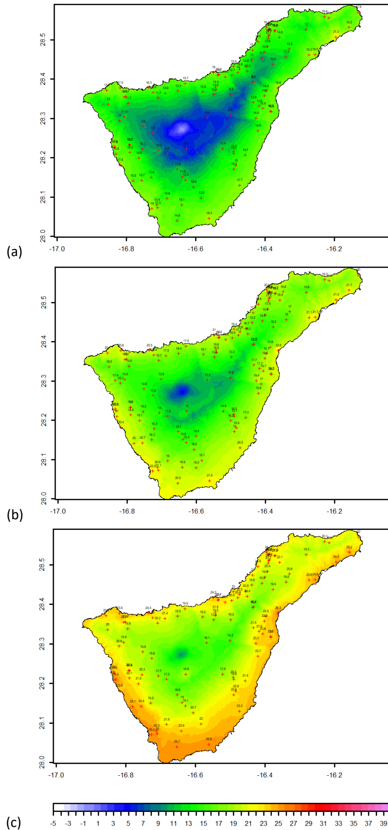
Figura 4.1.2. Mapas de temperatura de la isla de Tenerife a 100 m de resolución espacial promediados para el periodo 1991-2020. (a) Temperatura mínima, (b) Temperatura media y (c) temperatura máxima. Las cruces indican las posiciones de las estaciones meteorológicas utilizadas y los valores son las temperaturas medidas.
