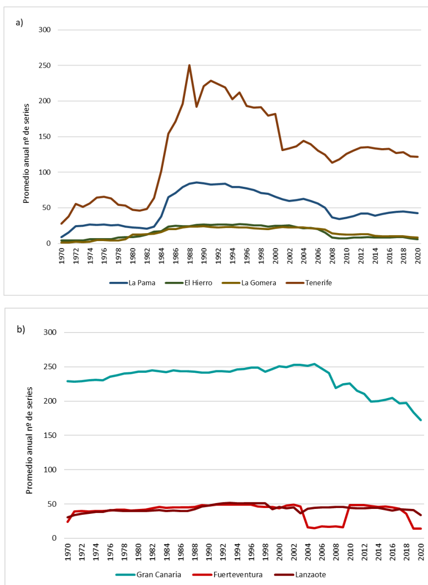
Figura 1.2.1. Promedio anual del número de series de precipitación en las islas occidentales (a) y en las orientales (b)
