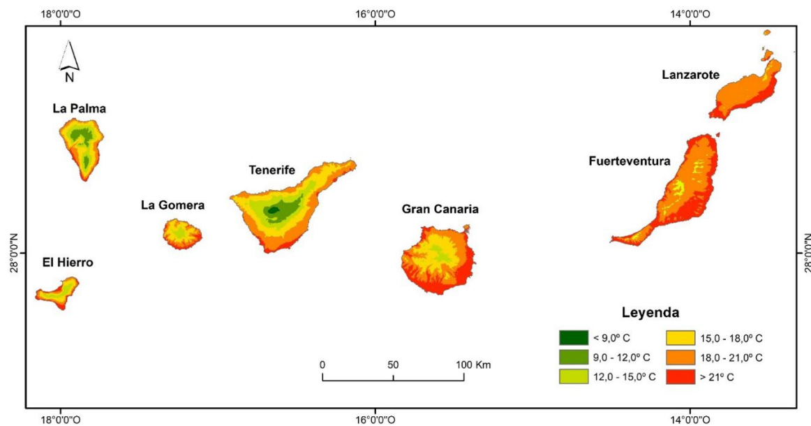
Figura 4.1.1 Temperatura media de Canarias promediada del periodo de 1991 a 2020. Mapas a 400 m de resolución espacial.
