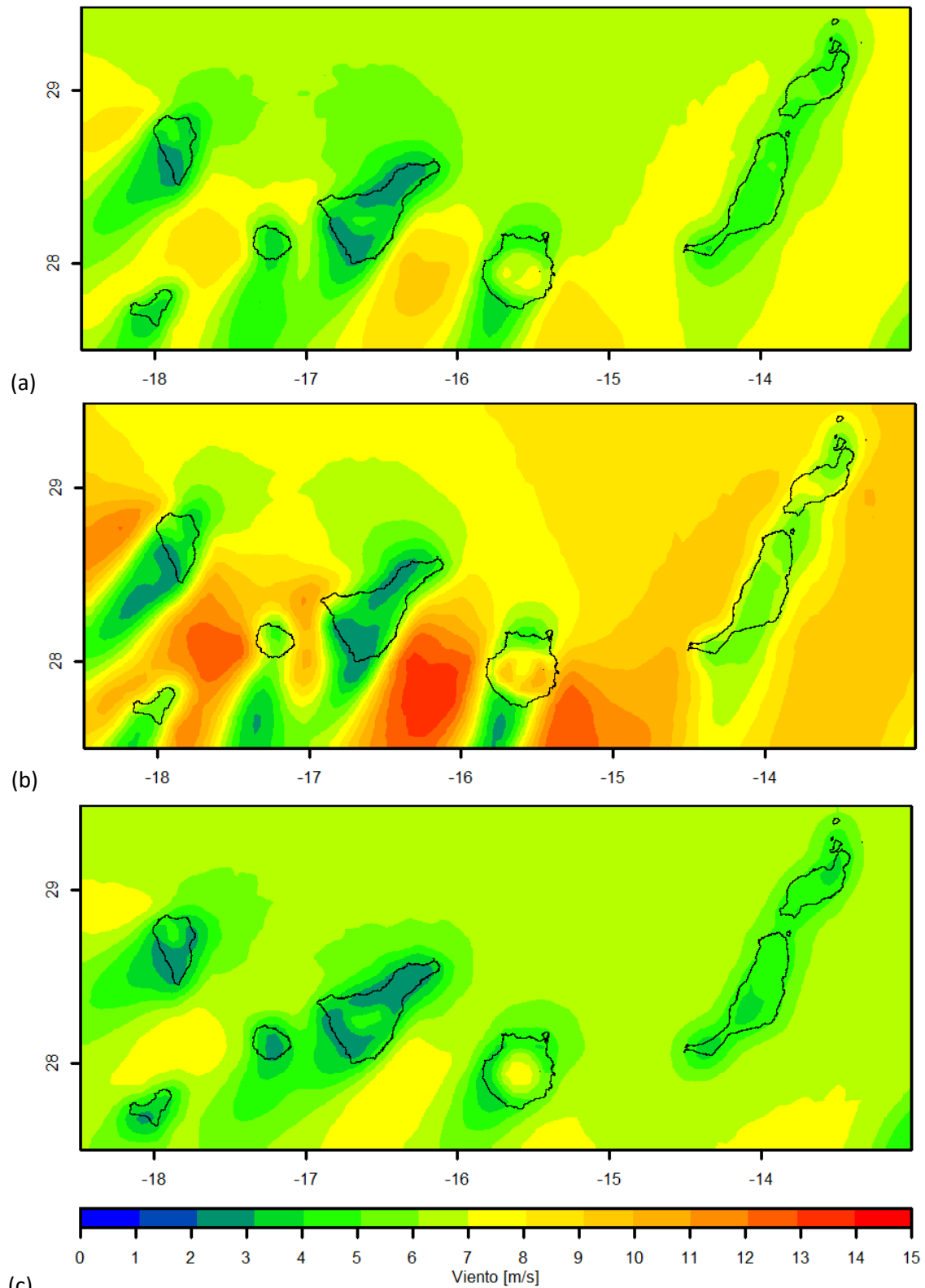
Figura 1.4. Viento del UERRA para archipiélago canario promediados desde el 2001 al 2020 a 400 m de resolución. (a) Promedio anual, (b) promedio de julio y (c) promedio de enero.
