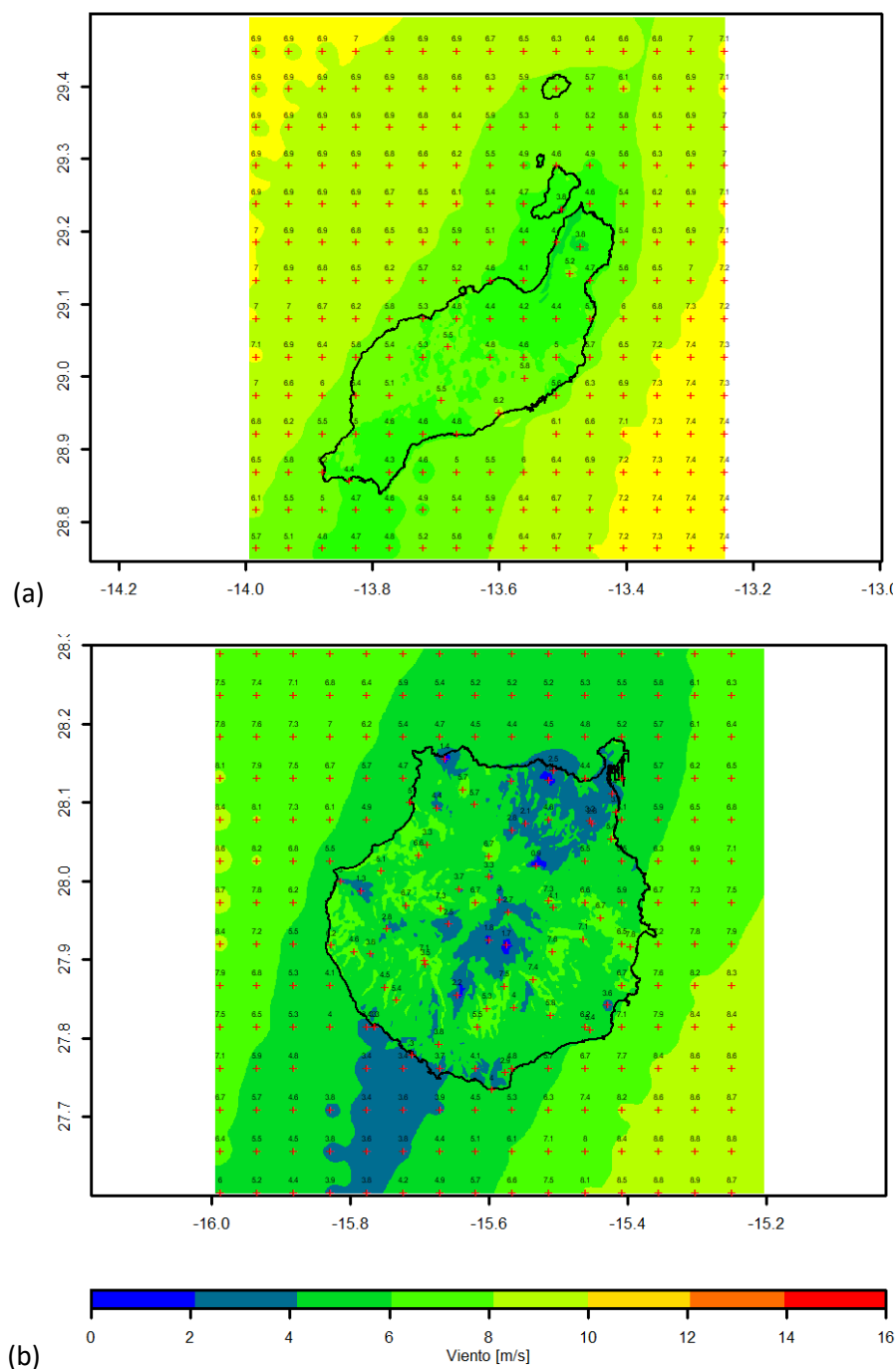
Figura 4.4.2. Mapas de intensidad de viento en m/s promediados entre 2001 y 2020 correspondiente a las islas de Lanzarote y Gran Canaria
