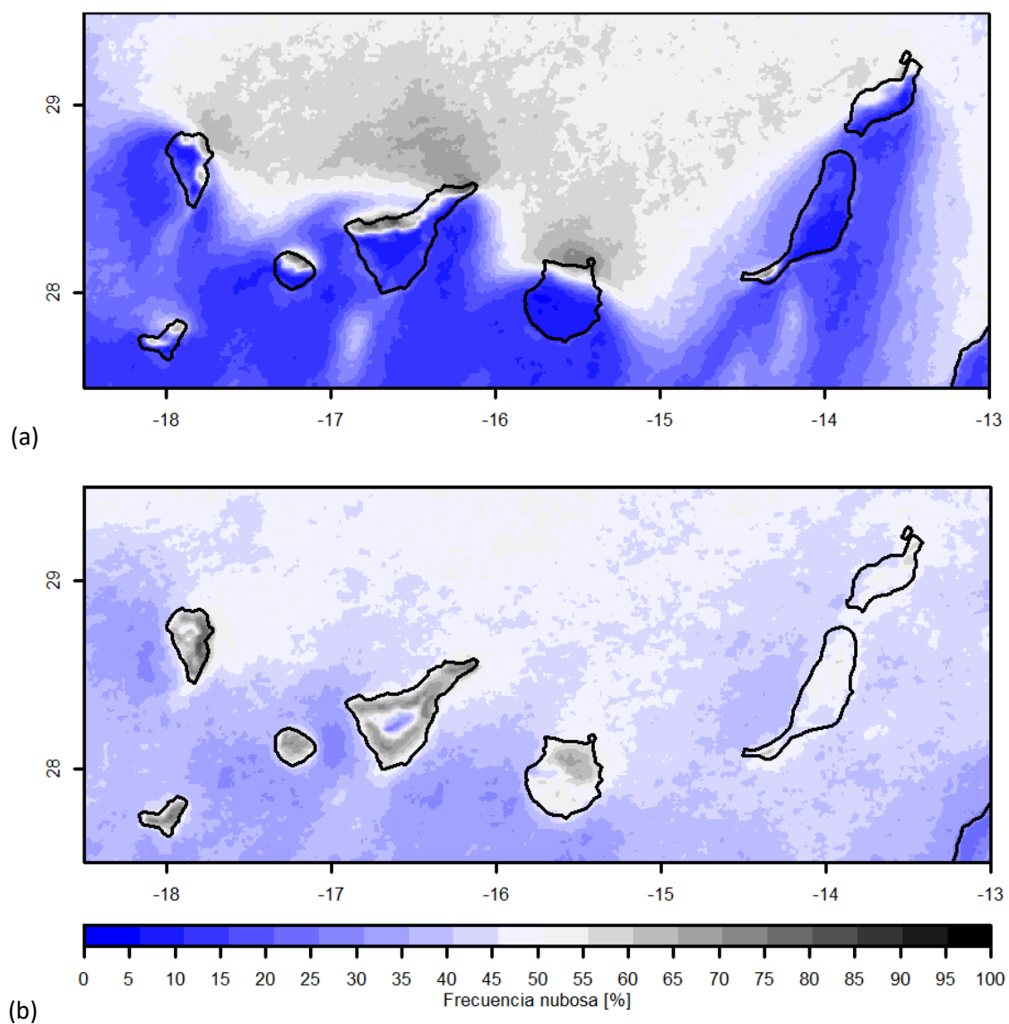
Figura 4.5.2. Frecuencia nubosa del mes de julio (a) y enero (b) a 400 m de resolución espacial promediada entre 2000 y 2014.
