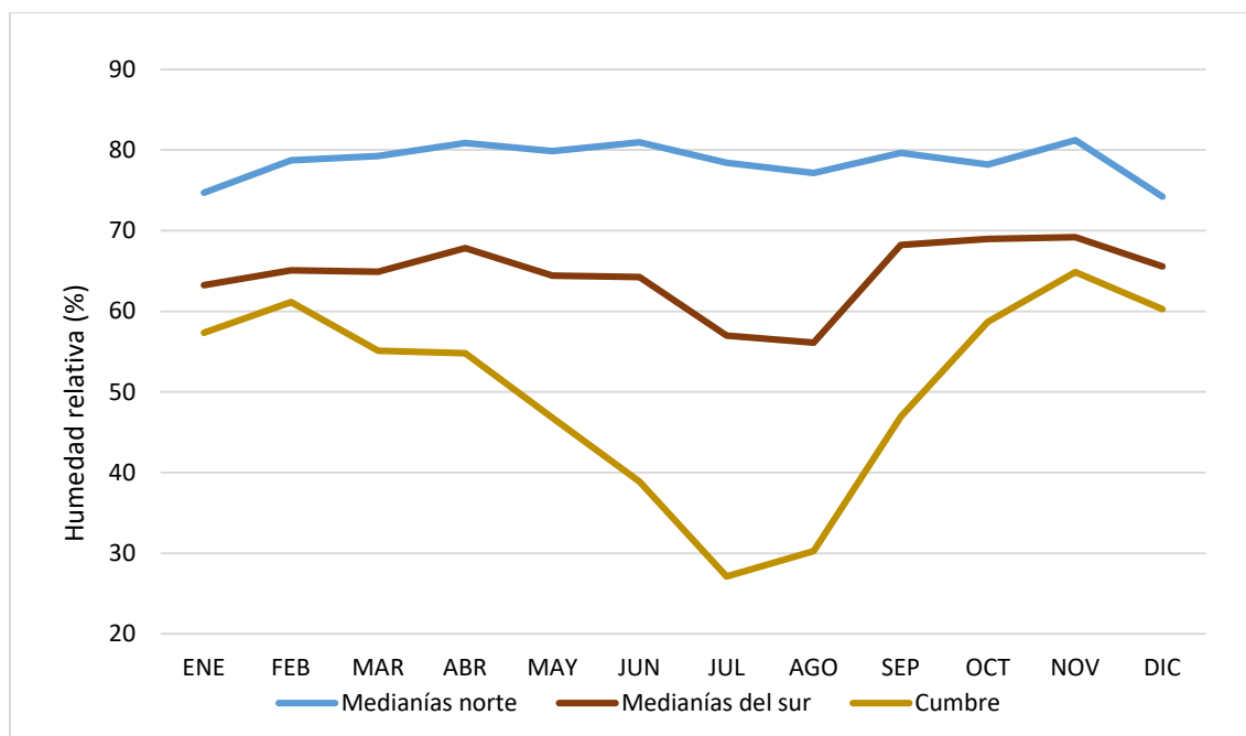
Figura 1.3. Humedad relativa mensual promedio en tres ámbitos diferentes del archipiélago.
