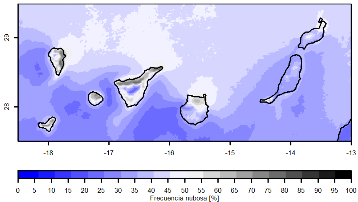
Figura 4.5.1. Frecuencia nubosa anual a 400 m de resolución espacial promediada entre 2000 y 2014.
