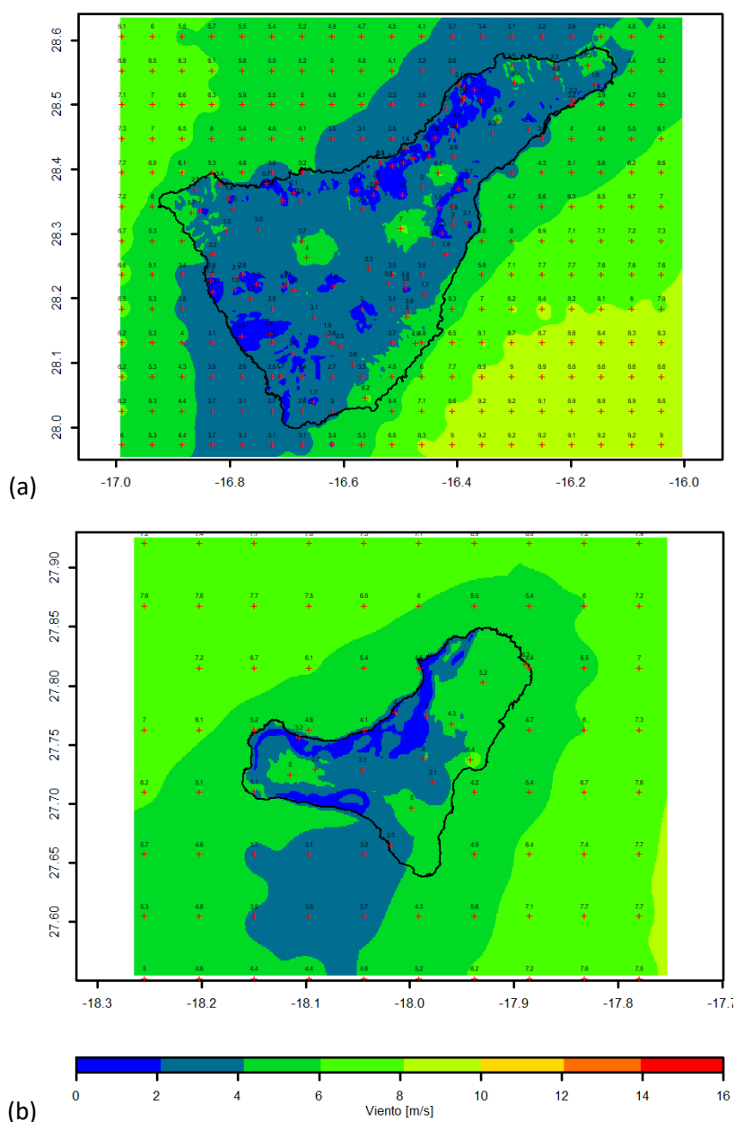
Figura 4.4.1. Mapas de intensidad de viento en m/s promediados entre 2001 y 2020 correspondiente a las islas de Tenerife y el Hierro.
