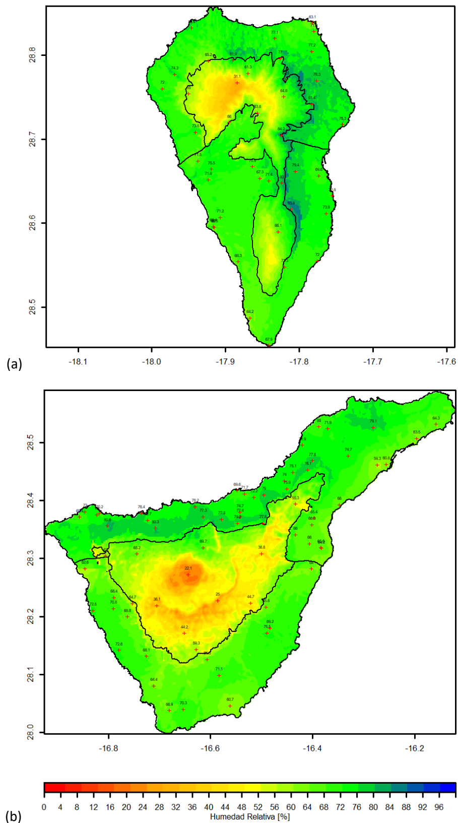
Figura 4.3.2. Humedad relativa a 100 m de resolución espacial promediados para el periodo 1991-2018 para la isla de La Palma (a) y entre 1991-2020 para la Isla de Tenerife (b). Las cruces indican las posiciones de las estaciones meteorológicas utilizadas y los valores numéricos son los valores promediados de las humedades de cada estación.
