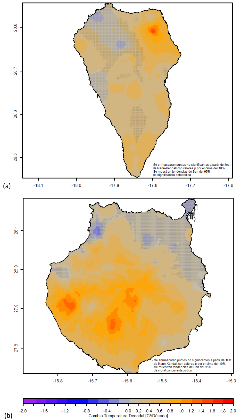
Figura 6.1 Tendencia decadal de temperatura en °C/década entre 1991 y 2020 para (a) La isla de la Palma y (b) La isla de Gran Canaria
