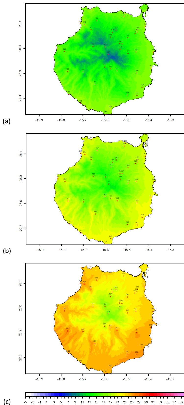
Figura 4.1.3. Mapas de temperatura de la isla de Gran Canaria a 100 m de resolución espacial promediados para el periodo 1991-2020. (a) Temperatura mínima, (b) Temperatura media y (c) temperatura máxima. Las cruces indican las posiciones de las estaciones meteorológicas utilizadas y los valores son las temperaturas medidas.
