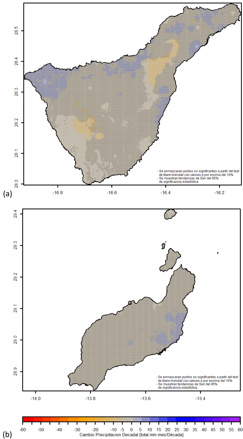
Figura 6.2 Tendencia decadal de precipitación en mm mes/década para (a) La isla de Tenerife entre 1986 2020 y (b) La isla de Lanzarote entre 1970 y 2020.
