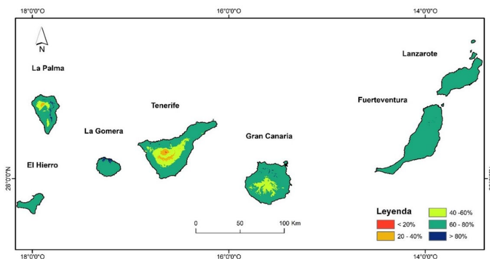
Figura 4.3.1. Humedad relativa promediada en el periodo 1991-2020 en Tenerife y Gran Canaria y 1991-2018 en el resto de islas a unos 400 m de resolución espacial.
