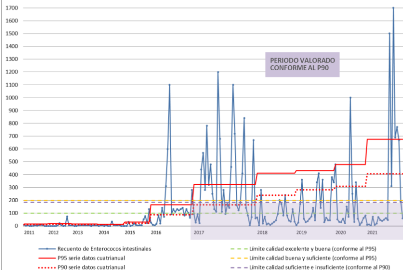
"PLAYA EL CONFITAL" PM1 - EVOLUCIÓN ENTEROCOCOS INTESTINALES (UFC/100ml) Temporadas de baño 2011-2021
