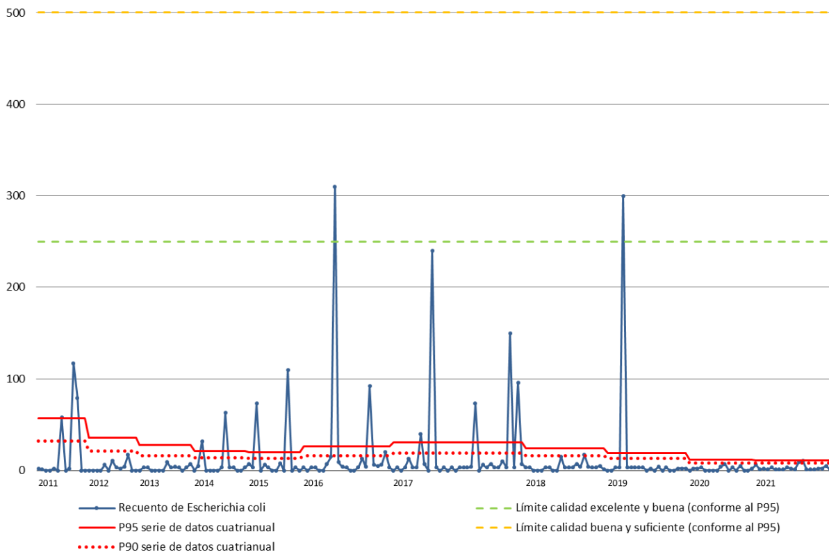
"PLAYA EL CONFITAL" PM1 - EVOLUCIÓN ESCHERICHIA COLI (UFC/100ml) Temporadas de baño 2011-2021
