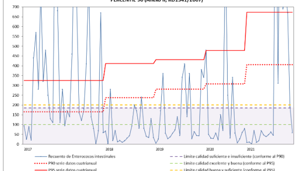
"PLAYA EL CONFITAL" PM1 - ENTEROCOCOS INTESTINALES PERIODO DE VALORACIÓN CONFORME AL PERCENTIL 90 (Anexo II, RD1341/2007)
