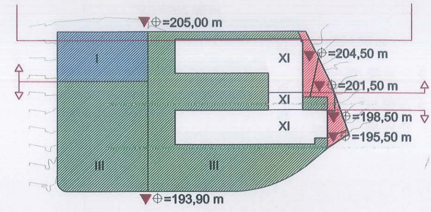
SECCIÓN LONGITUDINAL D-D'
