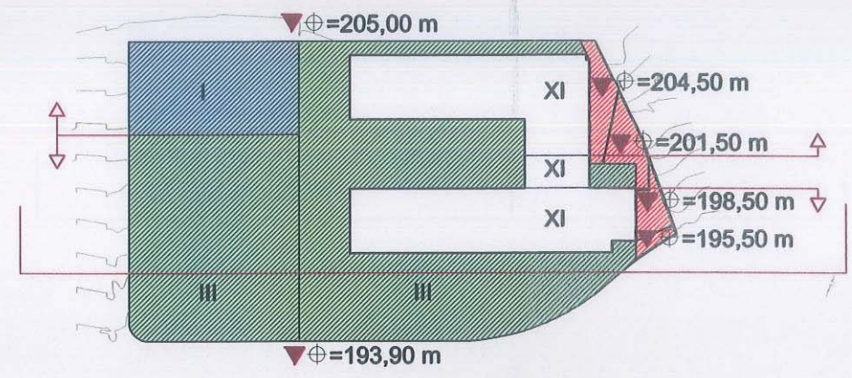
SECCIÓN LONGITUDINAL A-A'
