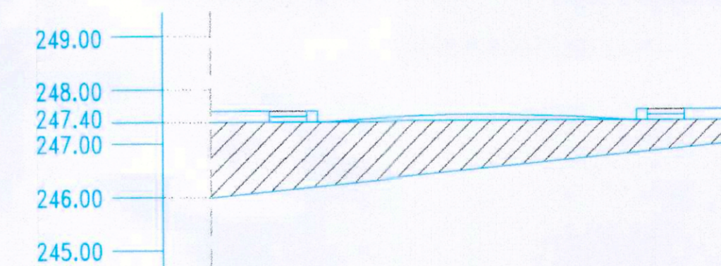
PERFIL TRANSVERSAL P-1 CALLE "H"
