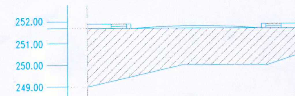
PERFIL TRANSVERSAL P-6 CALLE "G"
