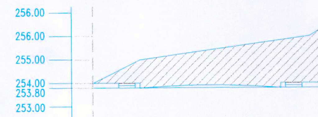
PERFIL TRANSVERSAL P-5 CALLE "G"
