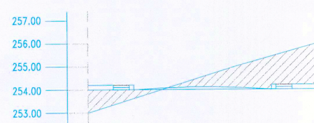
PERFIL TRANSVERSAL P-1 CALLE "G"
