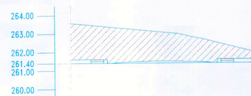
PERFIL TRANSVERSAL P-4 CALLE "F"
