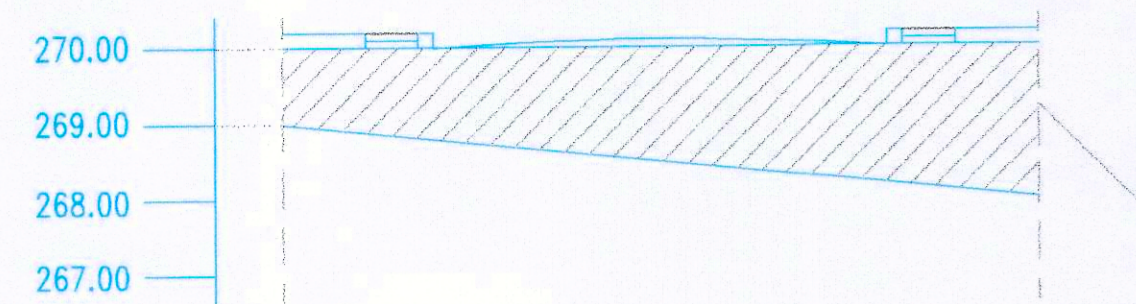
PERFIL TRANSVERSAL P-1 CALLE "F"
