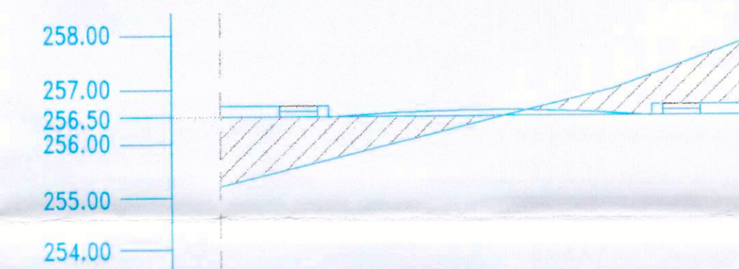
PERFIL TRANSVERSAL P-3 CALLE "G"
