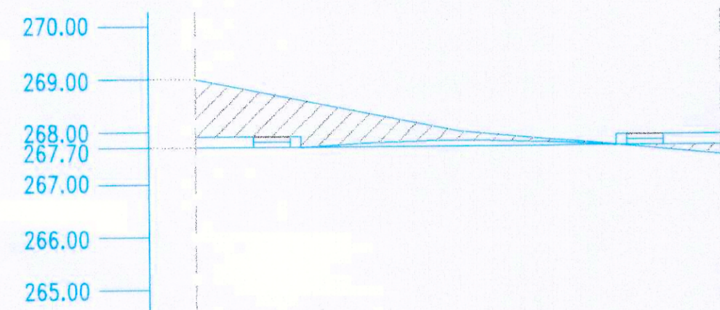
PERFIL TRANSVERSAL P-2 CALLE "F"
