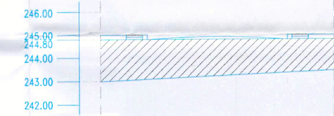
PERFIL TRANSVERSAL P-4 CALLE "H"
