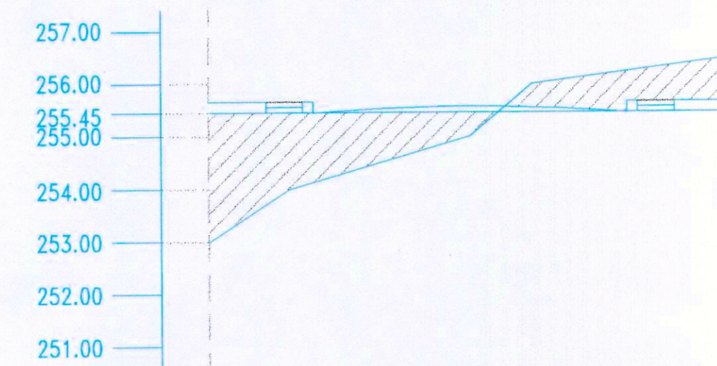
PERFIL TRANSVERSAL P-2 CALLE "G"
