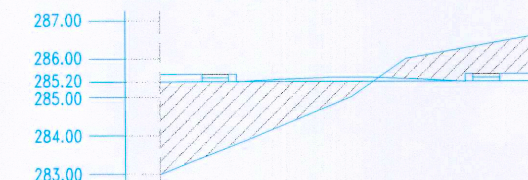
PERFIL TRANSVERSAL P-2 CALLE "D"
