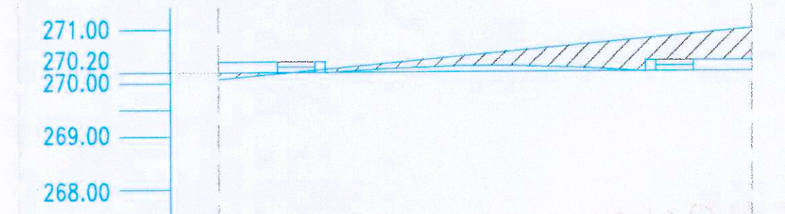
PERFIL TRANSVERSAL P-2 CALLE "E"
