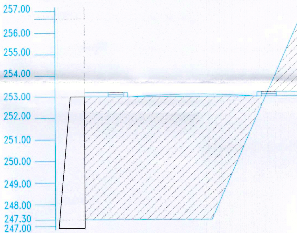
PERFIL TRANSVERSAL P-3 CALLE "C"
