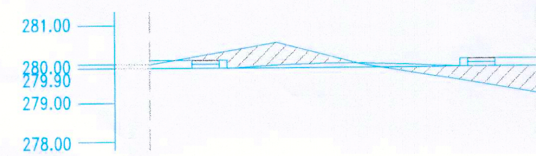
PERFIL TRANSVERSAL P-3 CALLE "B"
