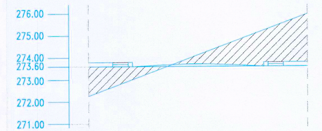
PERFIL TRANSVERSAL P-1 CALLE "E"
