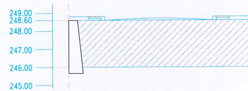
PERFIL TRANSVERSAL P-1 CALLE "C"
