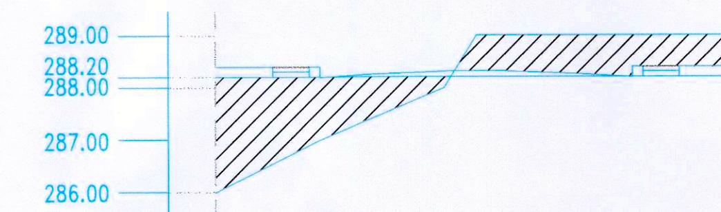
PERFIL TRANSVERSAL P-1 CALLE "D"
