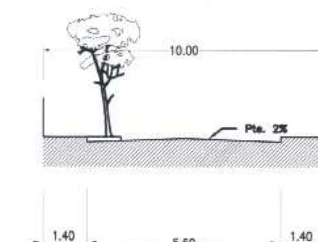
SECCION TIPO 2
