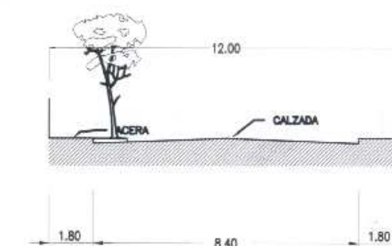
SECCION TIPO 1
