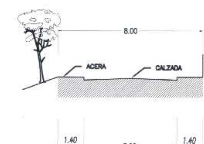
SECCION TIPO 3
