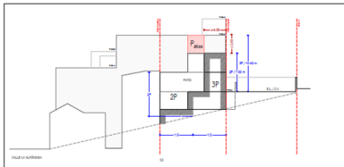
SECCIÓN TRANSVERSAL PARCELA 4 (C/ IMPERIAL, ESTRELLA Y VILLAVIEJA)
