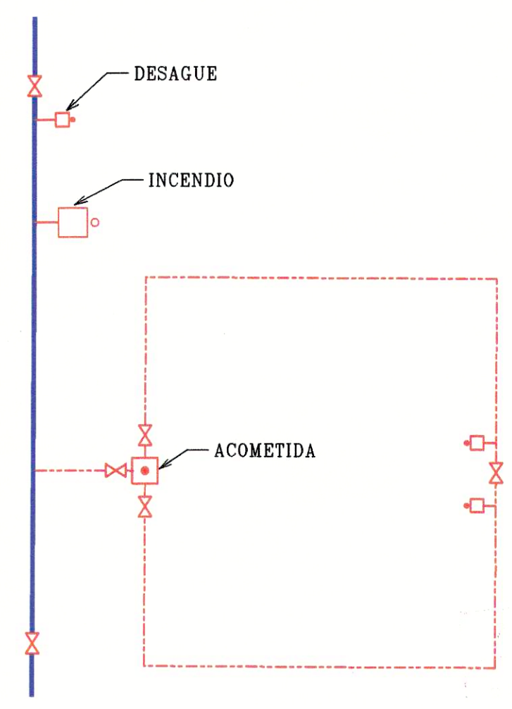
ESQUEMA DEL CIRCUITO CERRADO POR MANZANA
