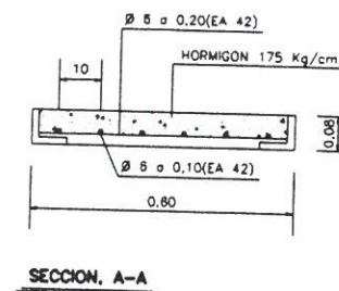
SECCION, A-A
