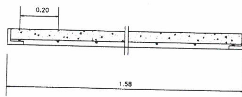
TAPA PARA ARQUETA DE VALVULA REDUCTORA DE PRESION
