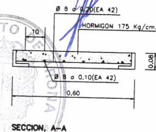
SECCION, A-A
