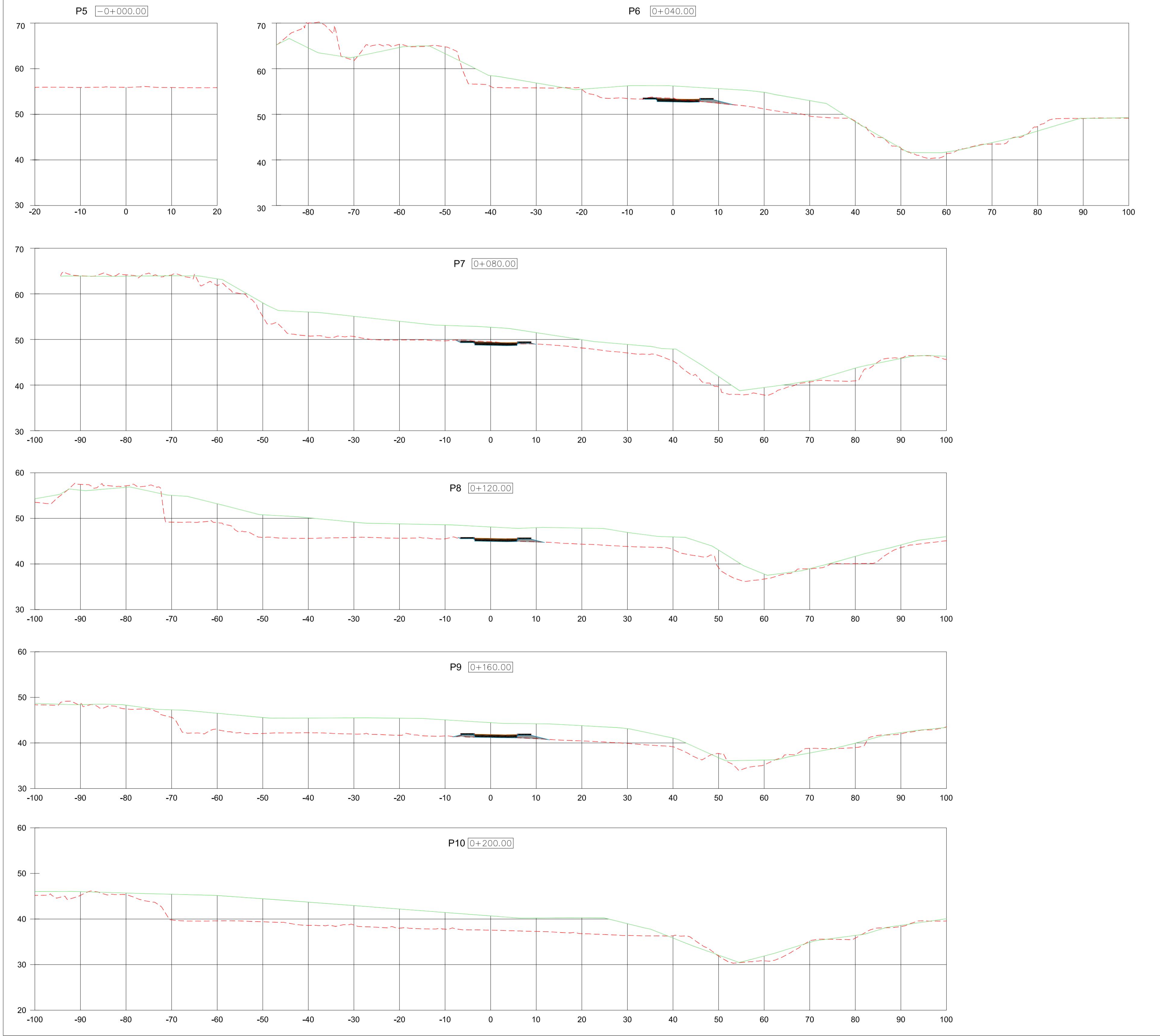
Perfiles transversales Vía de Distribución A y Parcelas 14 - 15
