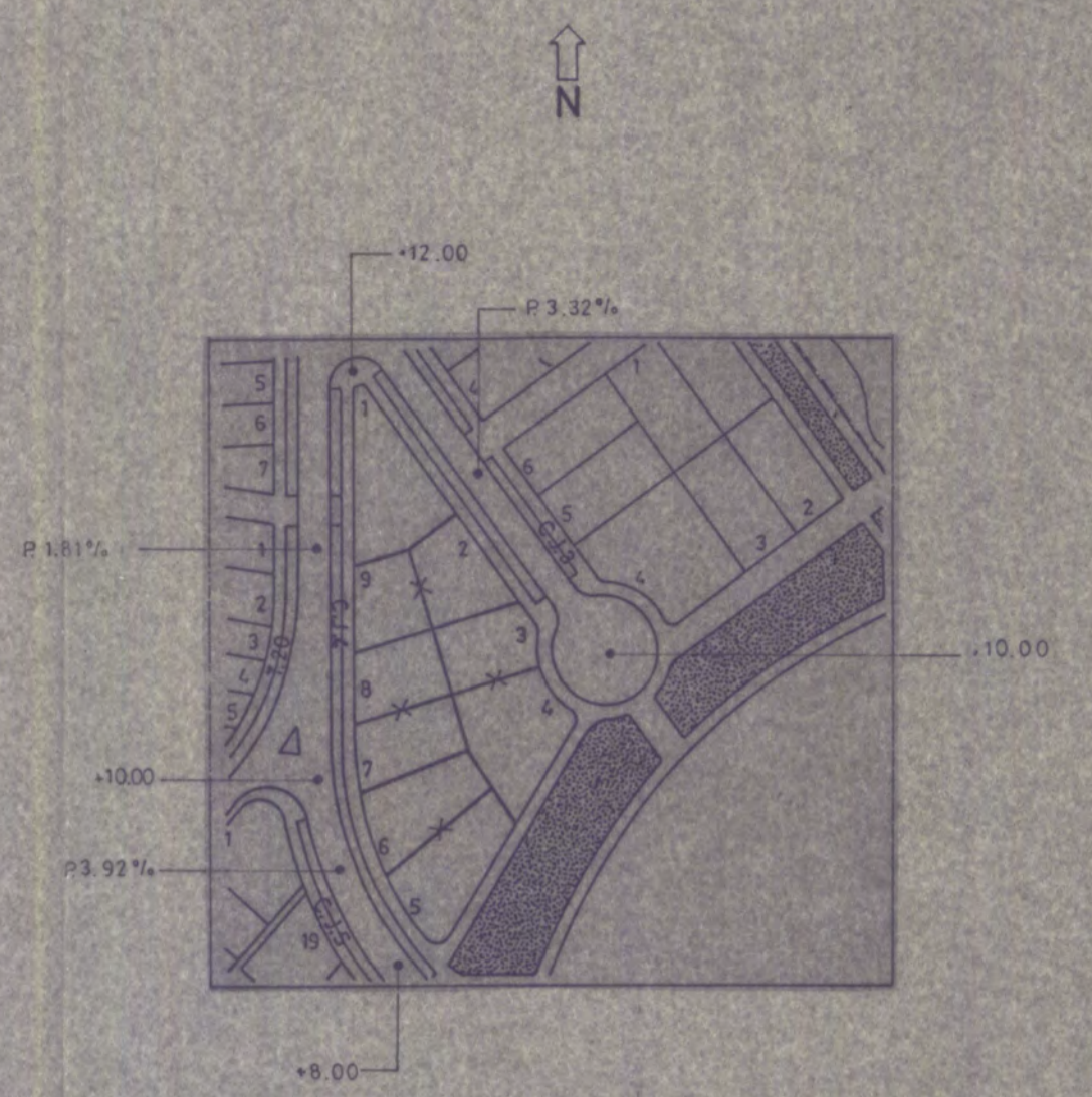
NIVELES Y RASANTES
