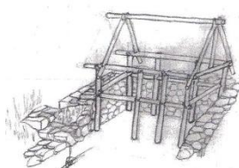
Armadura interna de madera de rollizos; Esteos, viga corredera, viga de la cumbrera, hibrones, palo de la cumbrera.
