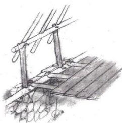
Armadura interna de madera; horcones, viga corredera, tiseras, suallado de tablas, viga de la cumbrera, hibrones.
