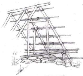
Armadura interna de madera del techo voladizo frontal.
