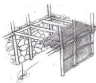
Armadura interna de madera; Esteos, viga corredera, tiseras, suallado de rollizos de falla o acebiño, cubierta de paja en los laterales, varas de acebiño en las paredes.
