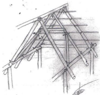
Armadura interna de madera de la cubierta; Cruceta, flechal, hibrones, palo de la cubierta, varas internas de acebiño.
