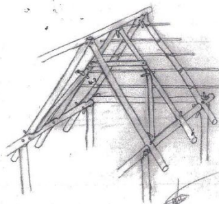
Armadura interna de madera de la cumbra; Cruceta, flechal, hibrones, palo de la cumbra, varas internas de acebiño.
