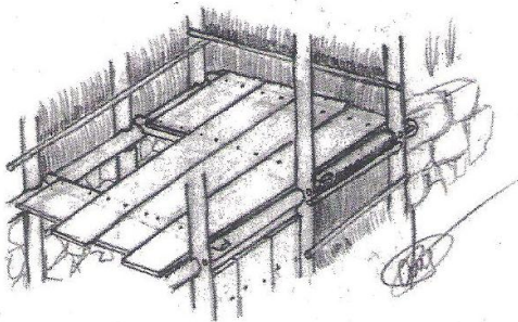
Armadura interna de madera; portillo en el suallado de madera
