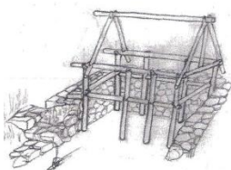
Armadura interna de madera de rollizos; Esteos, viga corredera, viga de la cumbrera, hibrones, palo de la cumbrera.
