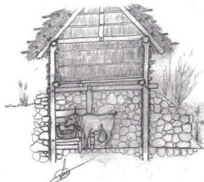
Armadura interna de madera; Corte interior frontal donde se visualiza todos los elementos de madera y colmo que componen una casa de cubierta vegetal.
