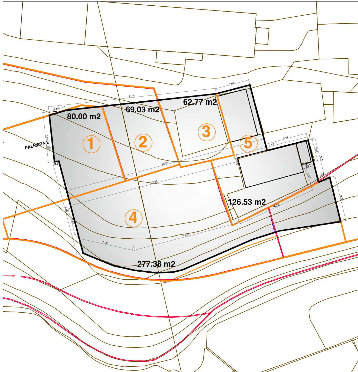
ESTRUCTURA DE LA PROPIEDAD. IDENTIFICACION DE LOS PROPIETARIOS EN EL AMBITO DE ORDENACION. ESCALA 1/250
