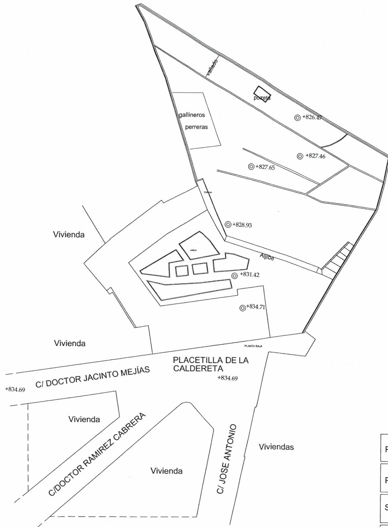
LEVANTAMIENTO TOPOGRÁFICO
