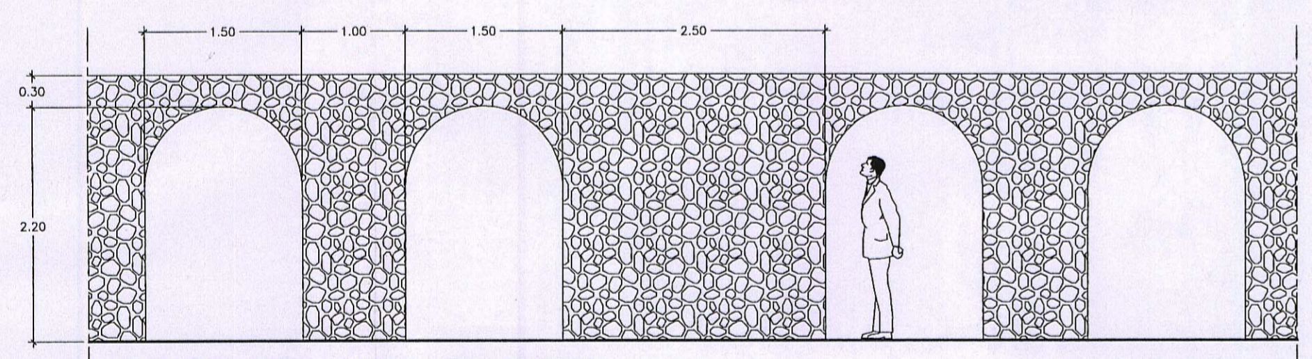
ALZADO TIPO MURO DE PIEDRA EN PASEO MARITIMO
