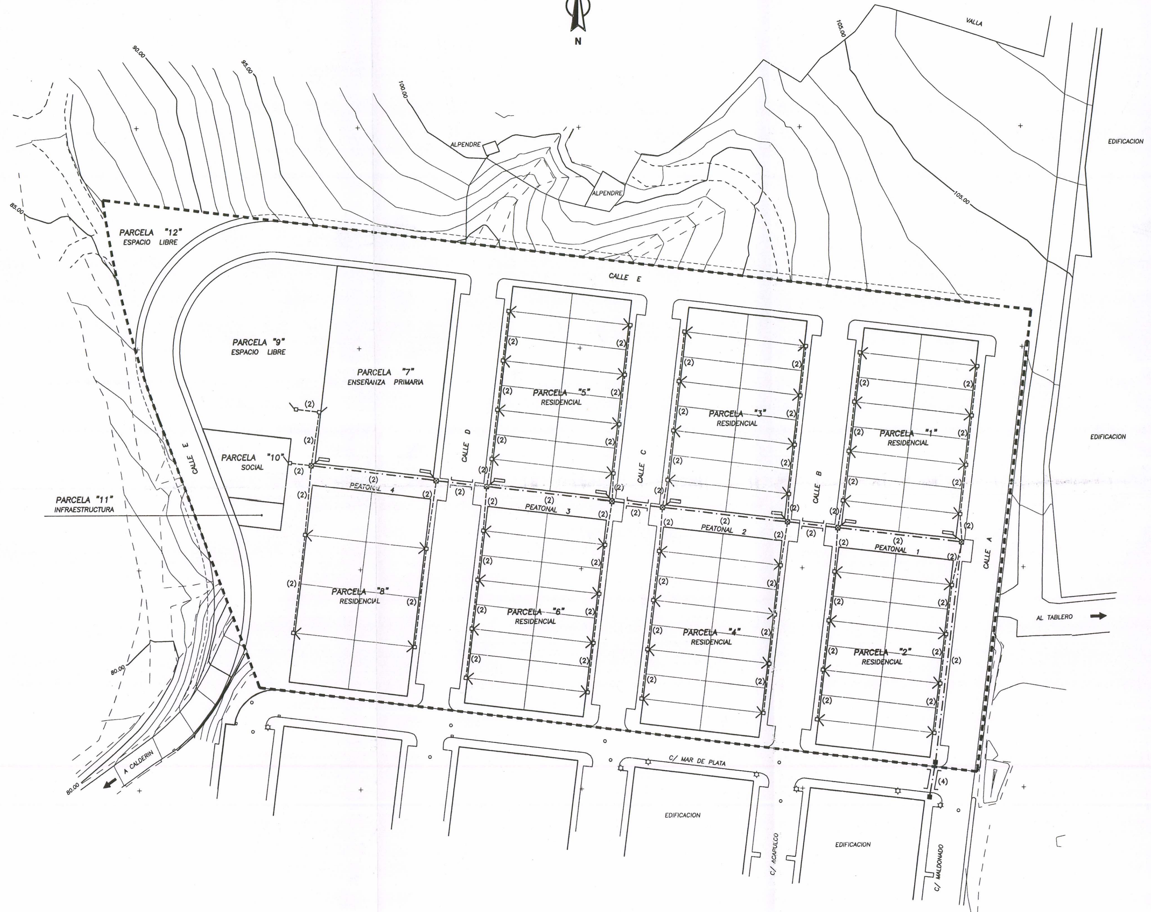
PLANTA GENERAL ESC: 1/500
