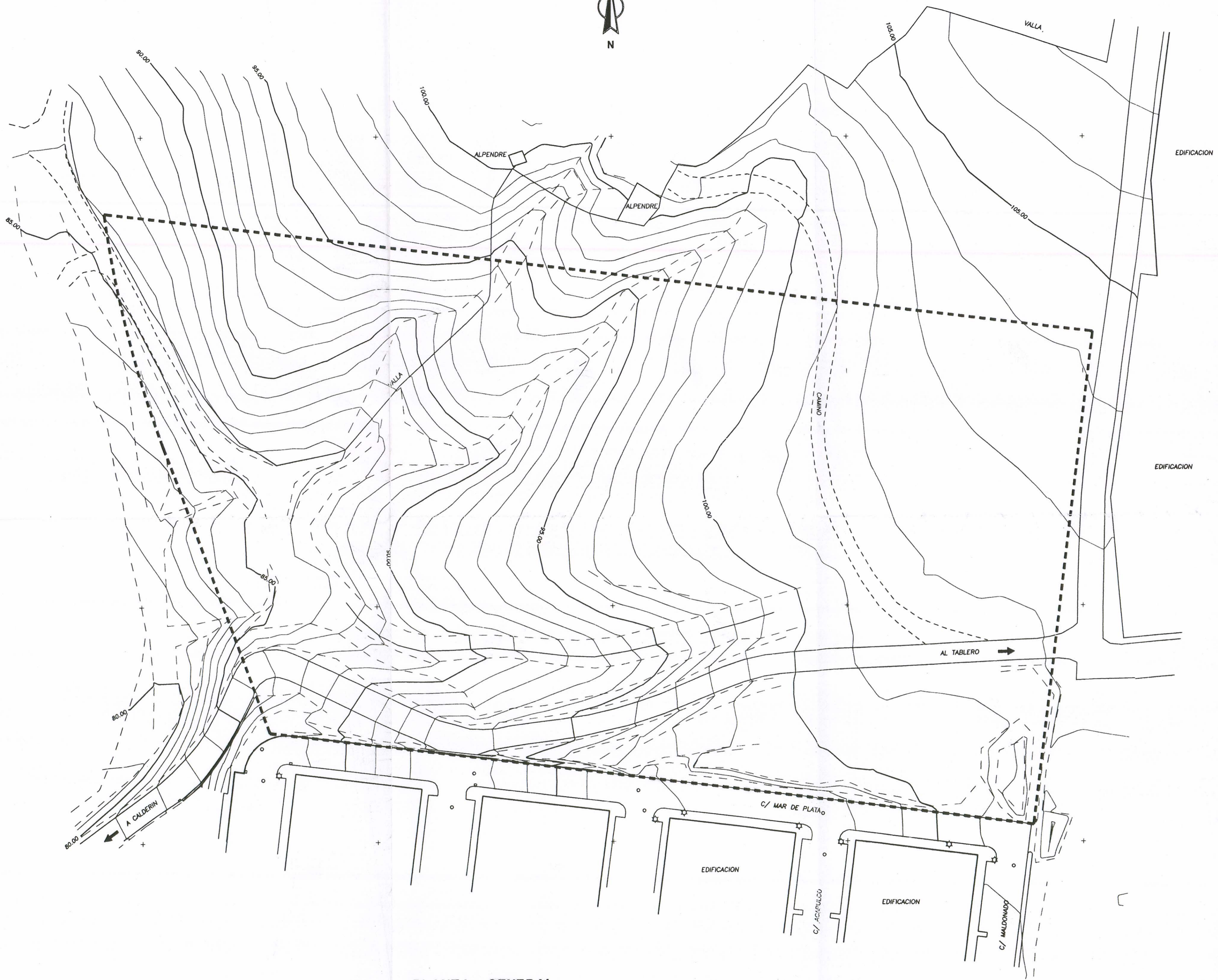
PLANTA GENERAL ESC: 1/500
