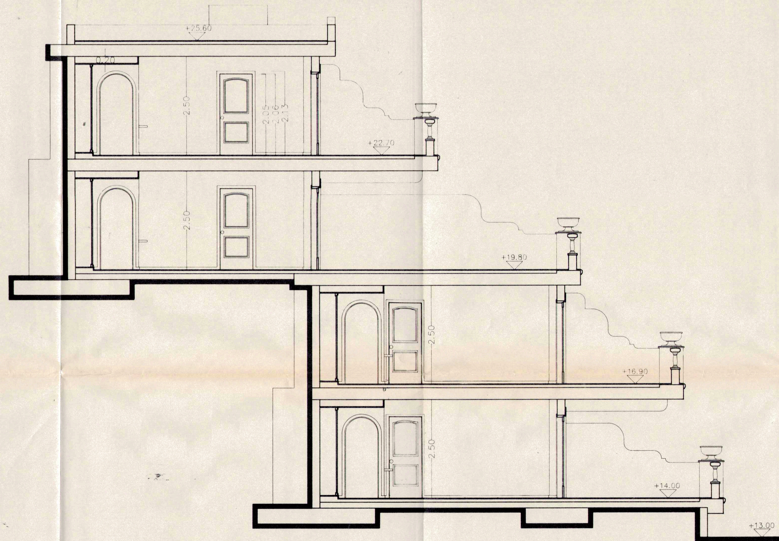
EDIFICIOS A y B SECCION GENERAL
