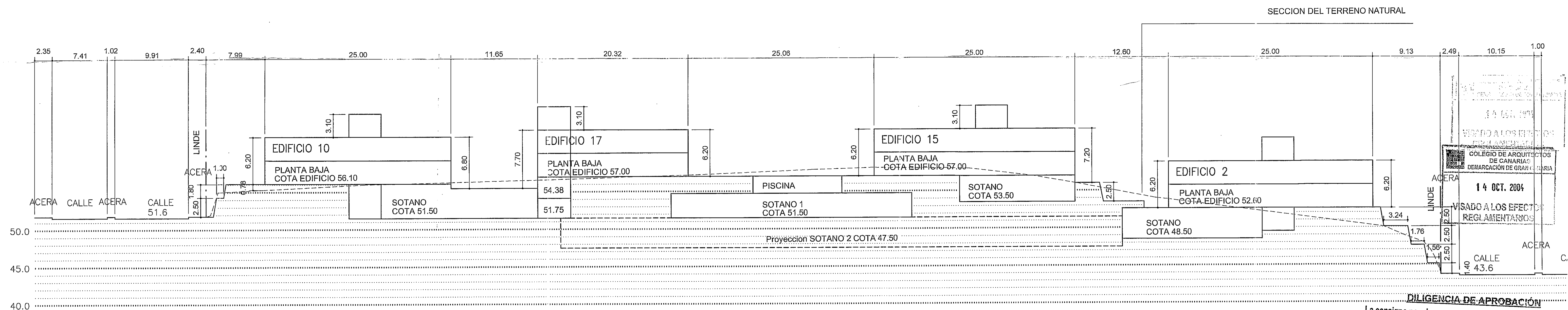
SECCION CC
