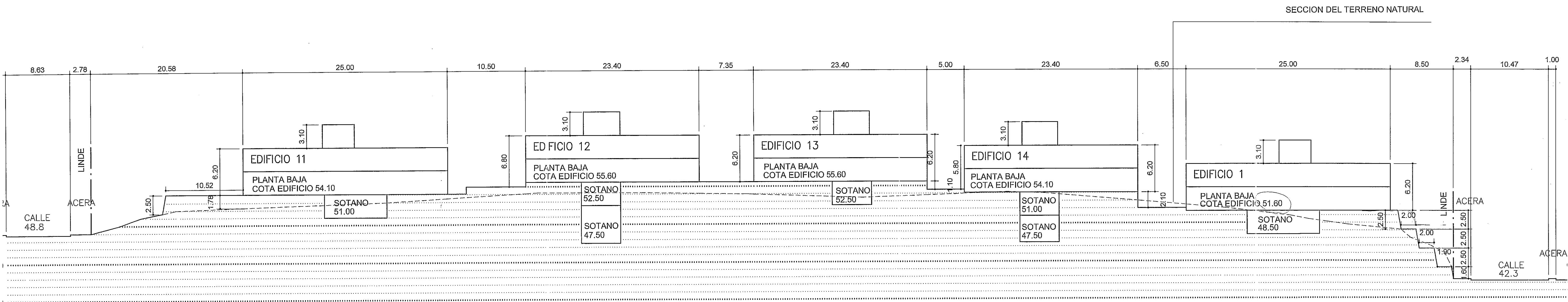
SECCION DD
