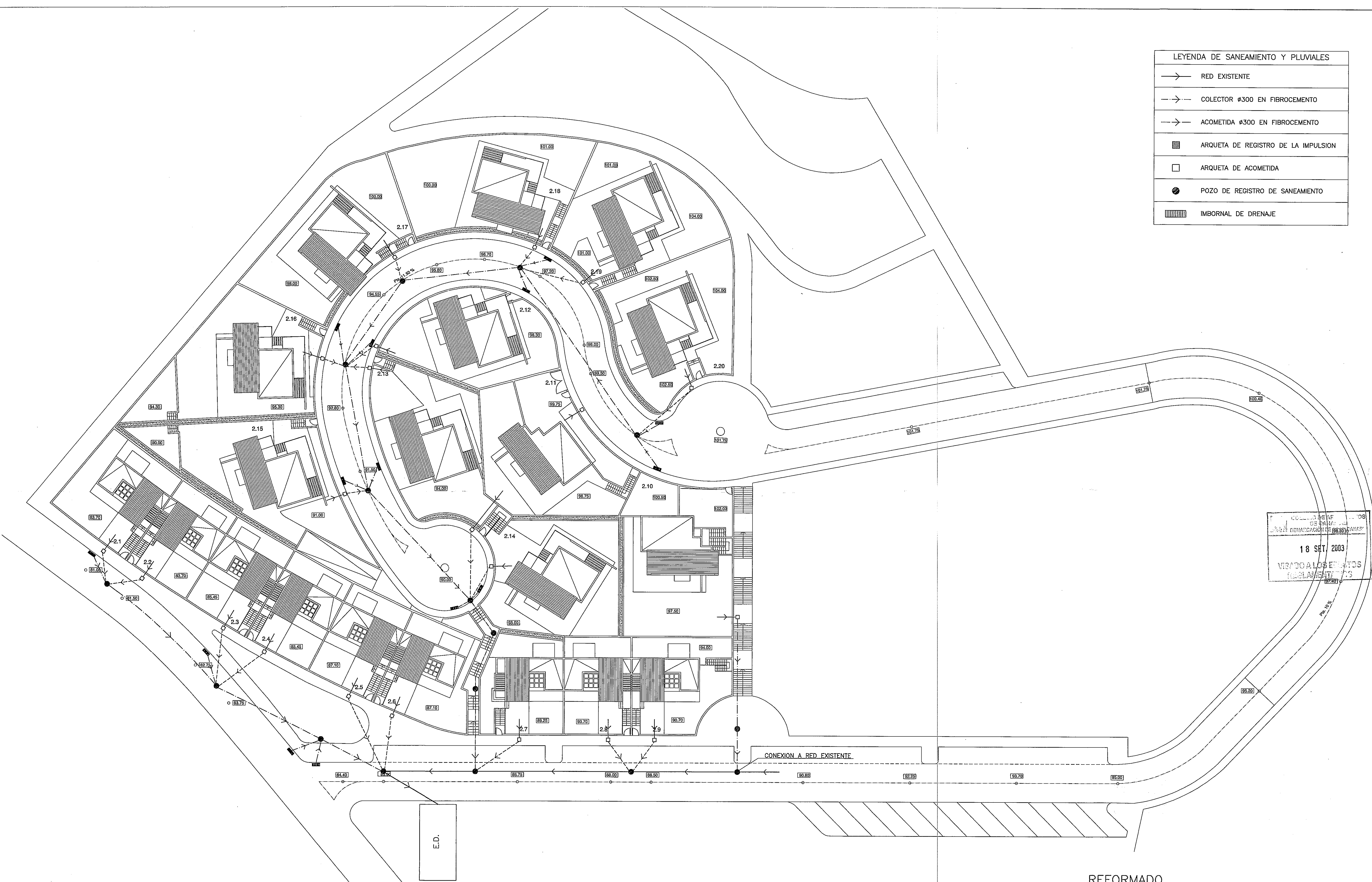
RED DE SANEAMIENTO Y PLUVIALES PARCELA Nº 2
