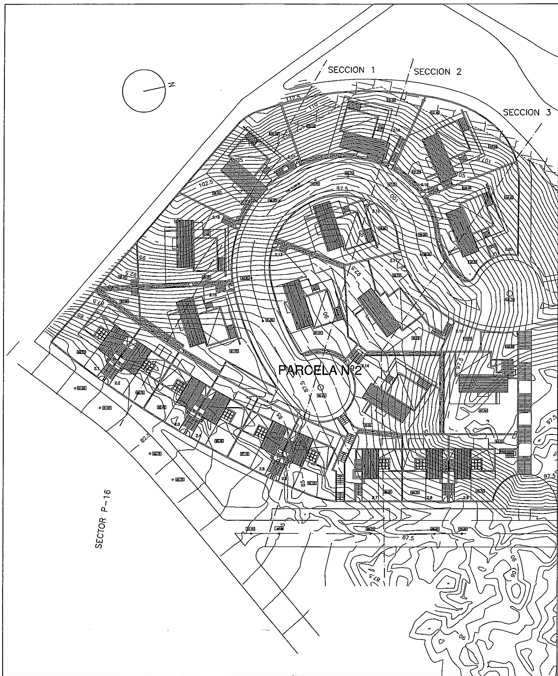
TOPOGRAFICO Esc. 1:500
