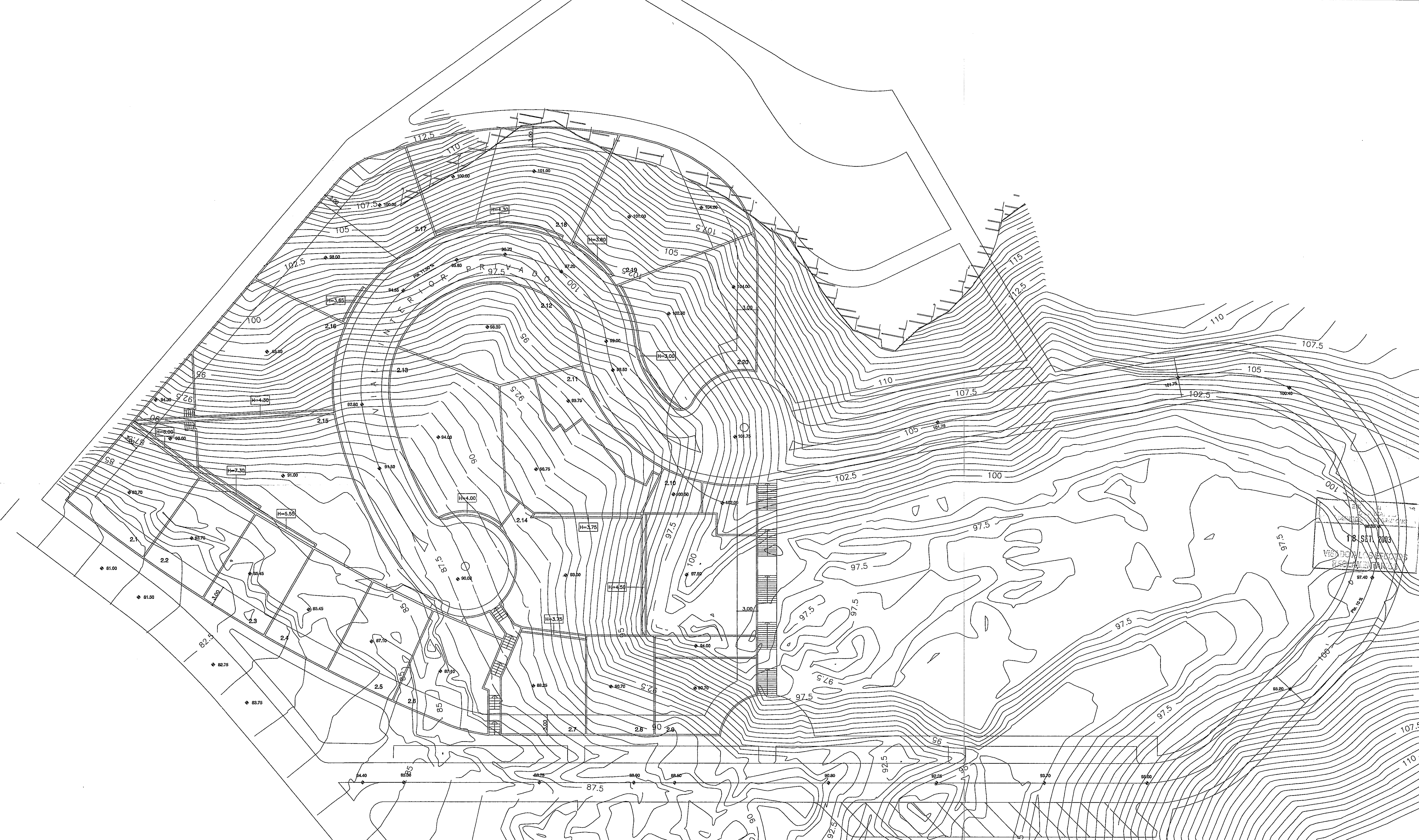
ALINEACIONES, RASANTES Y ALTURA DE MUROS PARCELA N° 2
