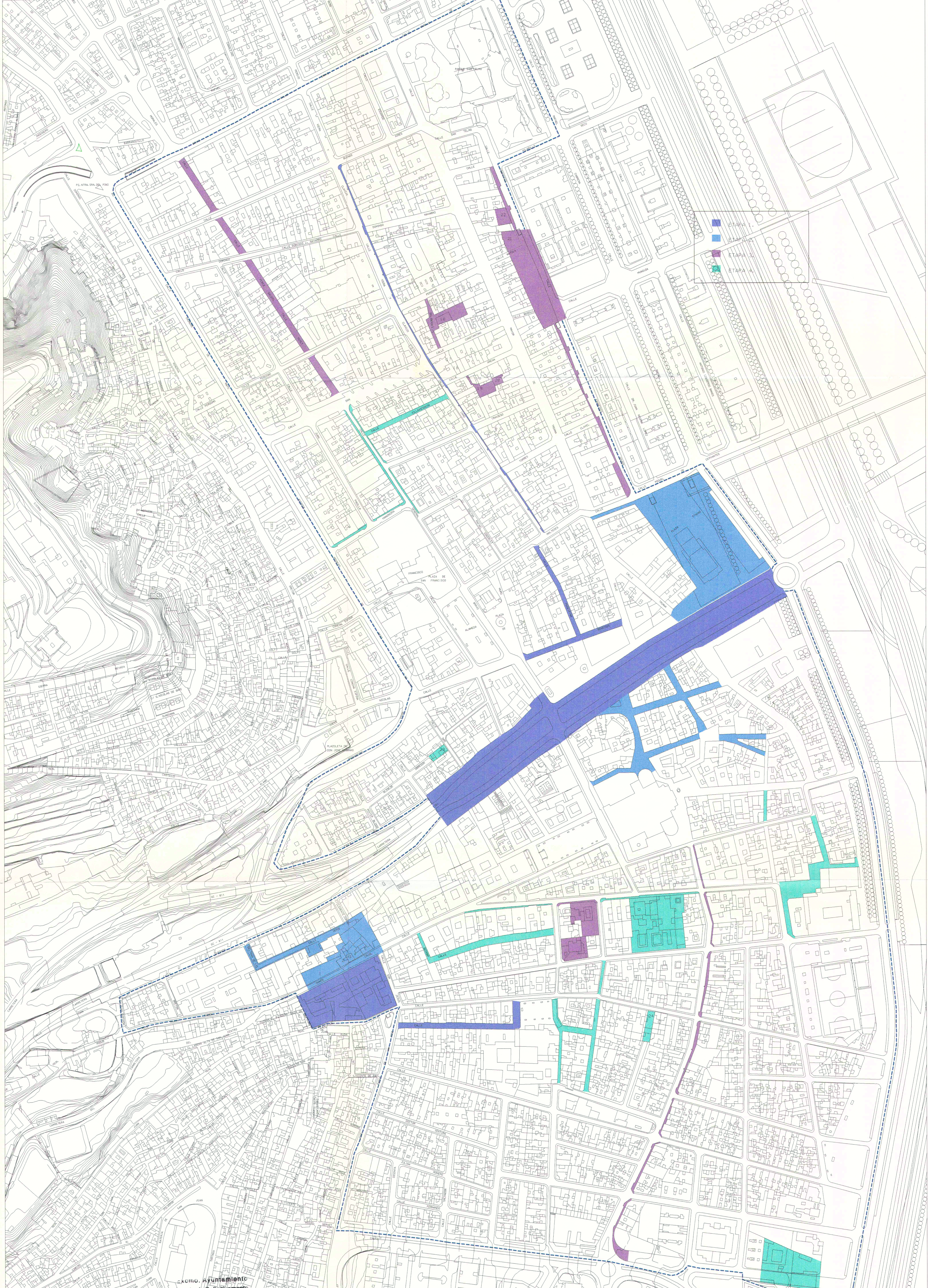
PLANO N. 7: PLAN DE ETAPAS. Escala 1/2.000.
