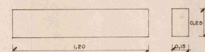
DETALLE DE BORDILLO EN CALZADA
