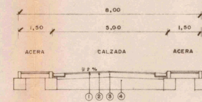
SECCION VIAL TIPO g
