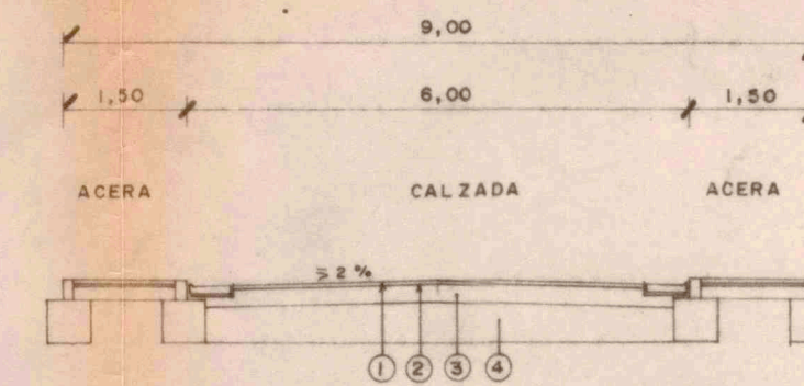
SECCION VIAL TIPO f
