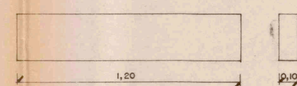
DETALLE DE BORDILLO EN ACERA
