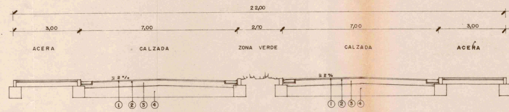
SECCION VIAL TIPO a
