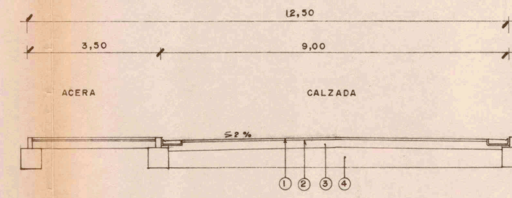
SECCION VIAL TIPO d'
