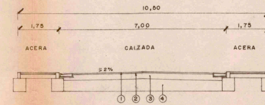
SECCION VIAL TIPO e
