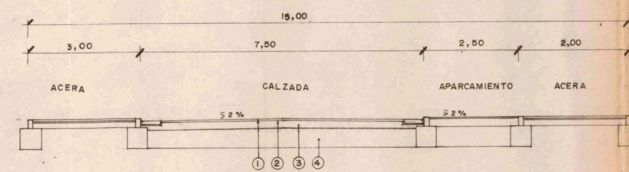
SECCION VIAL TIPO d
