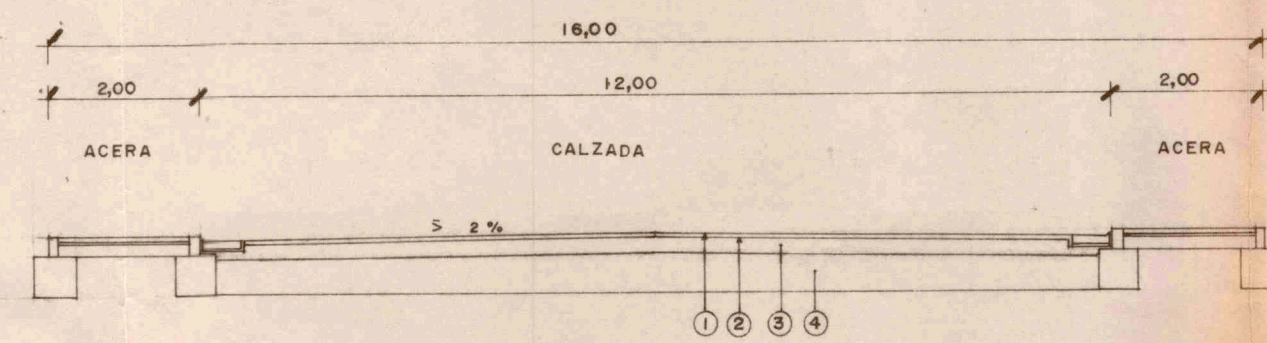
SECCION VIAL TIPO b
