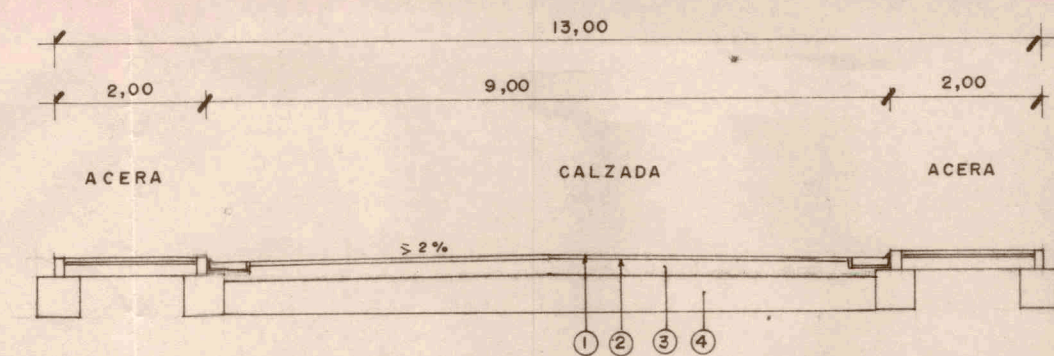
SECCION VIAL TIPO c
