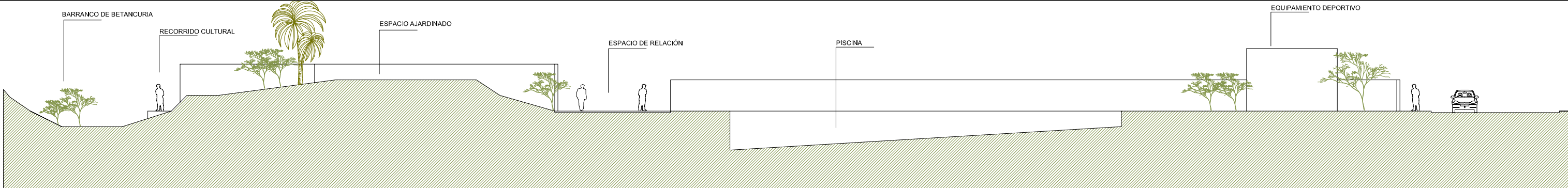
SECCIÓN LONGITUDINAL. EQUIPAMIENTO DEPORTIVO-PISCINA (d-d')
