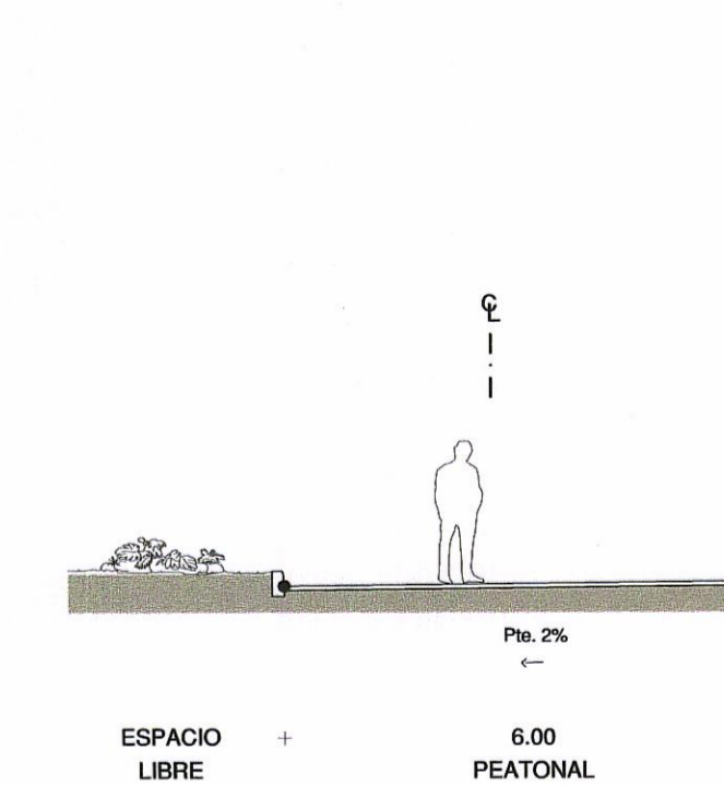
PEATONAL "J" 6.00 m.
