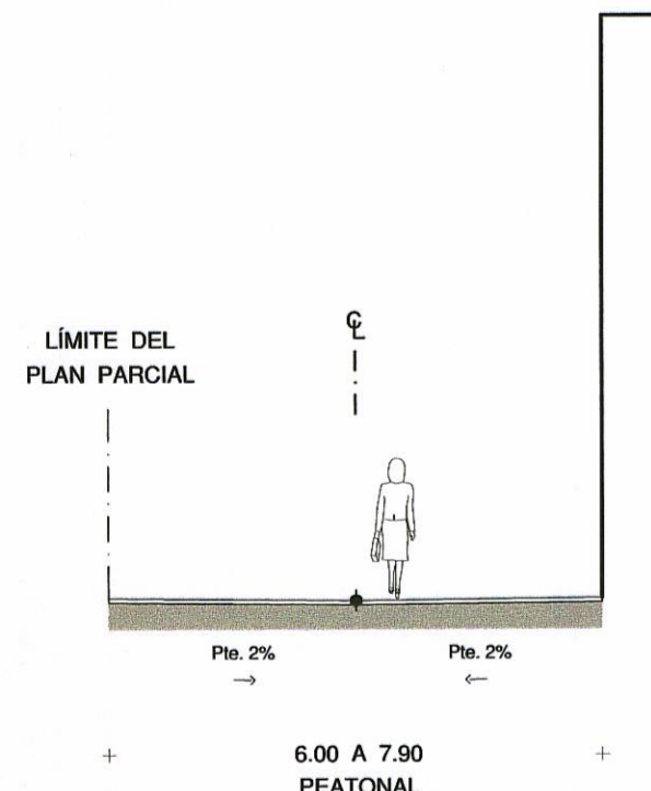
PEATONAL "B" 6.00 A 7.90 m.
