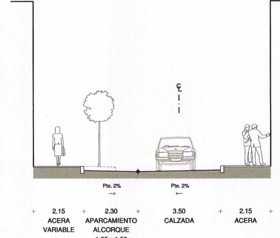
CALLES "G, H y P" 10.10 m.
