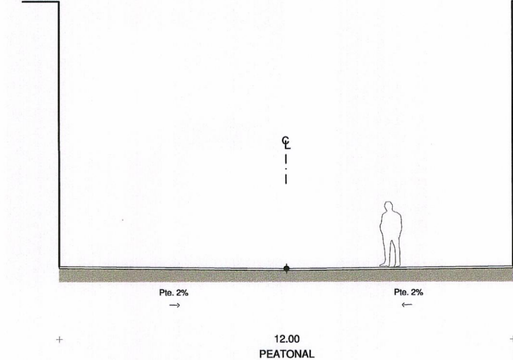
PEATONALES "E, O y Q" 12.00 m.
