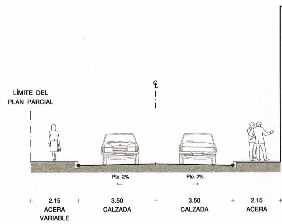
CALLE "A" 11.30 m.
