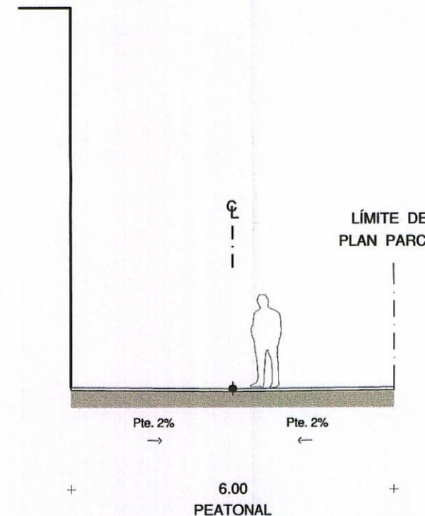
PEATONAL "F" 6.00 m.
