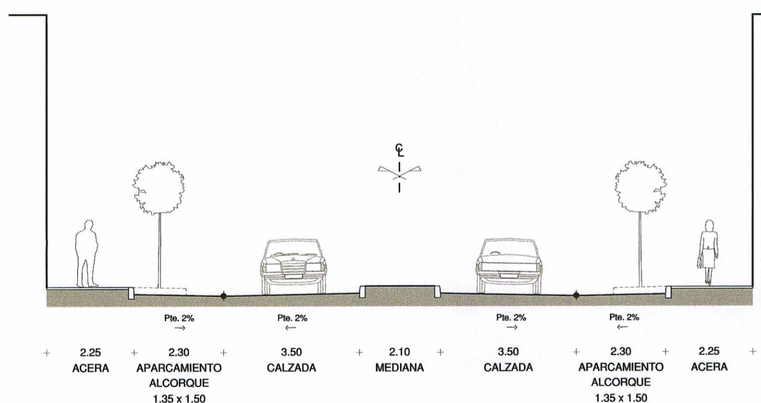
CALLE "R" 18.20 m.
