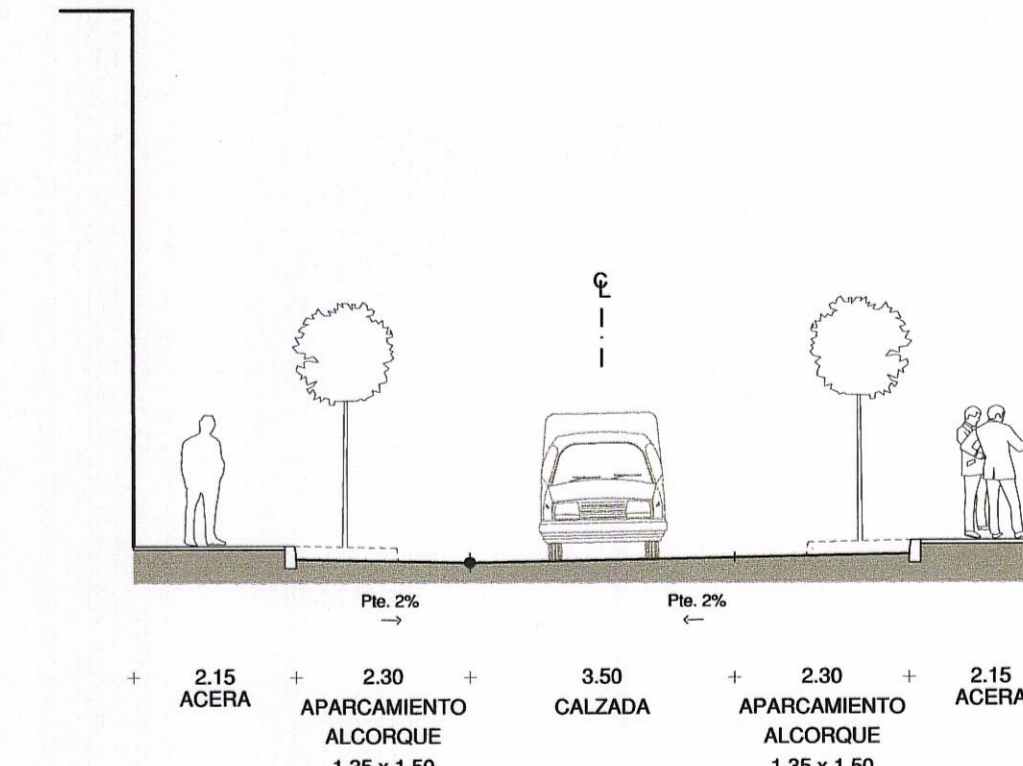
CALLES "D, G, K, y N" 12.40 m.
